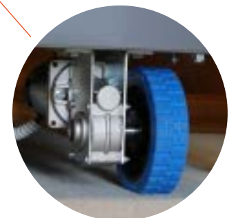
Motore elettrico a lunga durata con ruota motorizzata integrata Ø150mm
